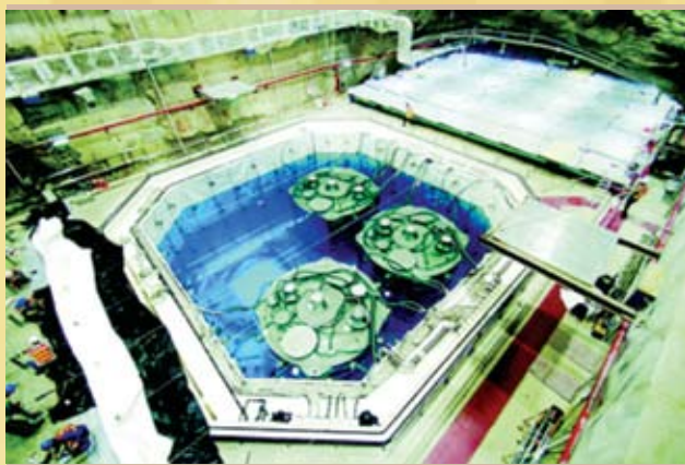
大亚湾实验发现中微子新的振荡模式
